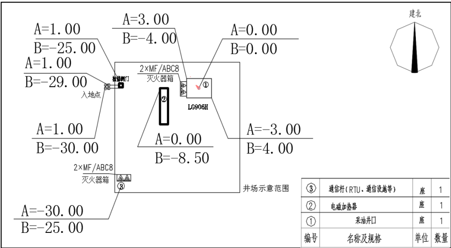
3.4-3 运营期井场平面布置示意图
