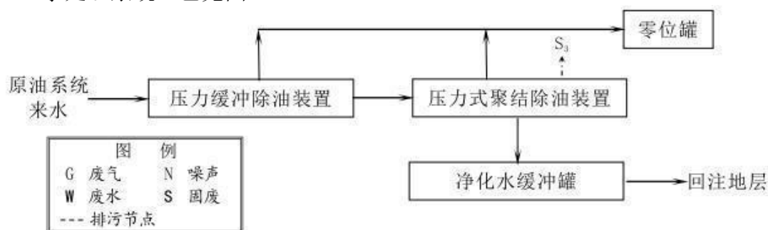
图 3.2-3 水处理系统工艺流程图
