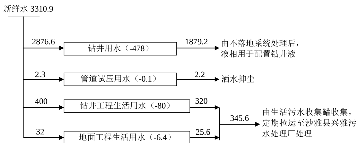
图 3.4-4 项目施工期给排水平衡图 (单位: \text{m}^3 )
