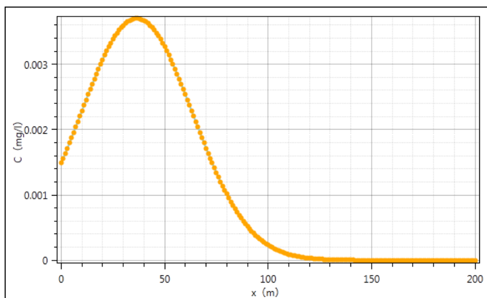
图 5.4-3 施工期石油类运移结果图
