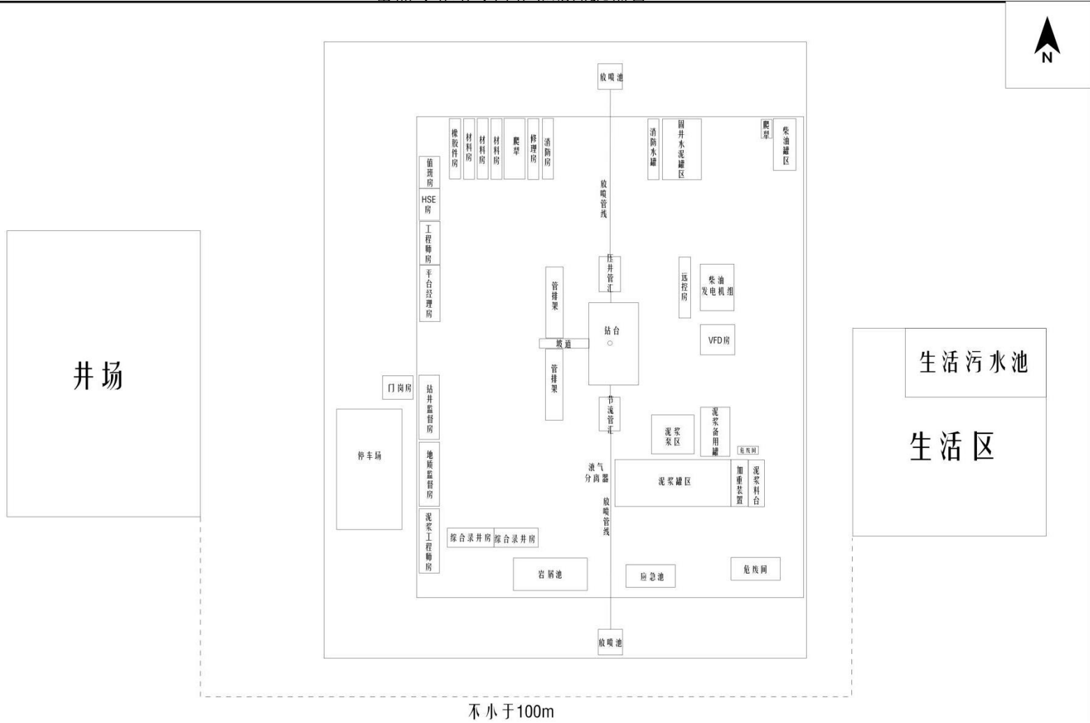
图 3.4-2 钻井期井场平面布置示意图
