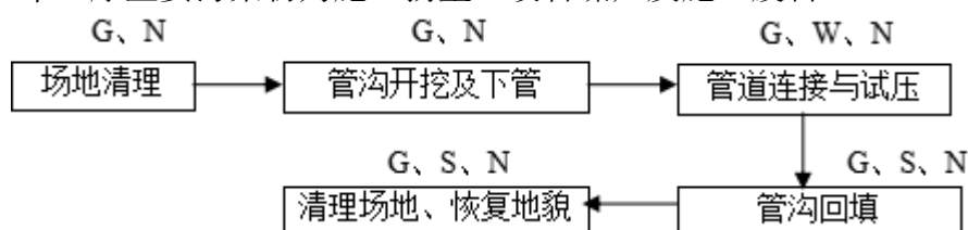
图 3.4-9 油气集输工程工艺流程及排污节点图
