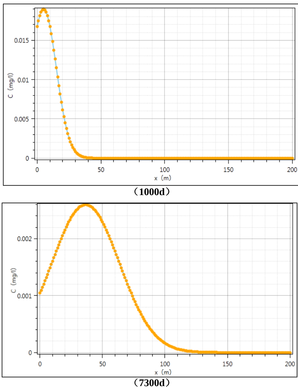
图 5.4-4 运营期石油类运移结果图
