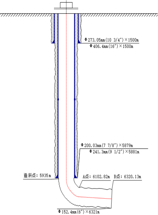
图 3.4-1 井身结构图
