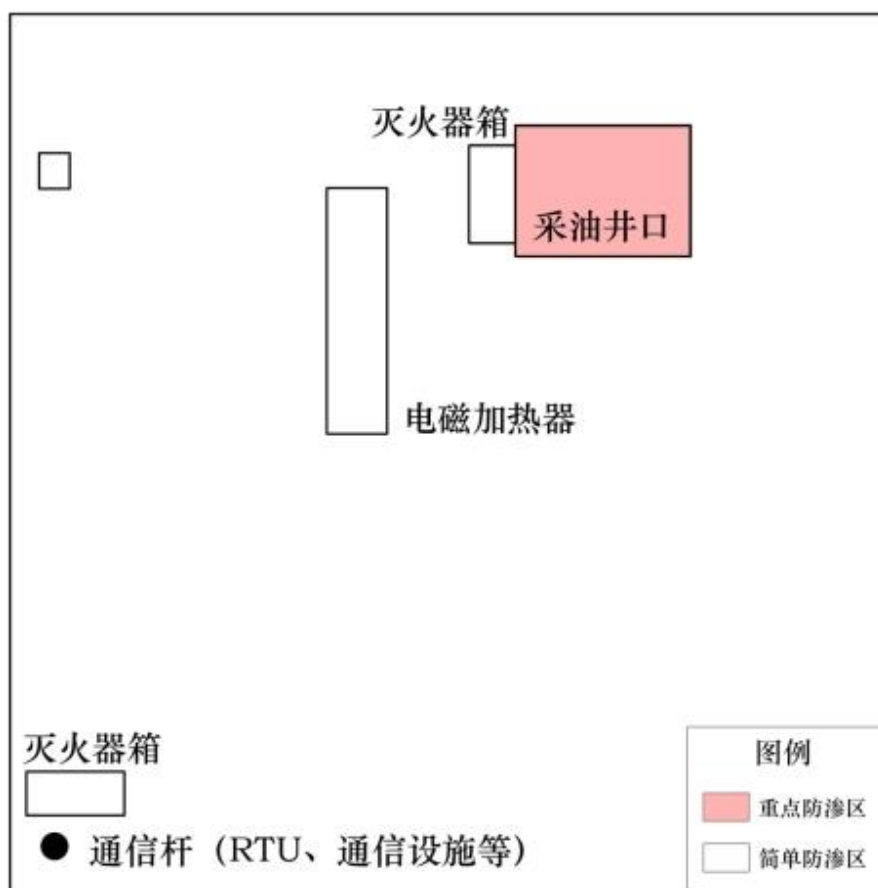
图5.4-6 运营期防渗分区图
